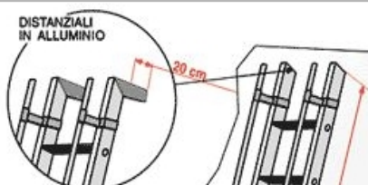
distanziali in alluminio saldati
